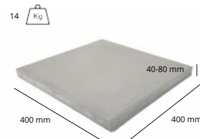
Le socle convient pour 12 dalles de 40 à 40 cm
