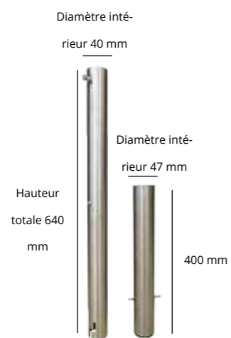
Ancrage au sol
