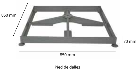
Pied de dalles
