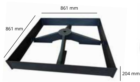
Pied de dalles
