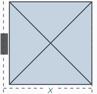
PALESTRO PRO 300X400 X=3140 MM PALESTRO PRO 400X400 X=4140 MM
