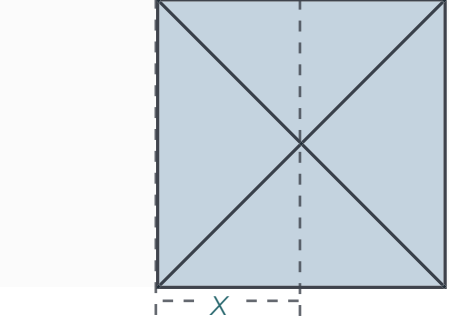
BASTO PRO 400X400 X=2000 MM BASTO PRO 500X500 X=2500 MM
