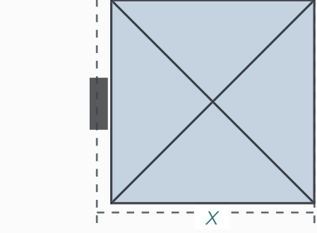
PALESTRO PRO 300X400 X=3140 MM PALESTRO PRO 400X400 X=4140 MM
